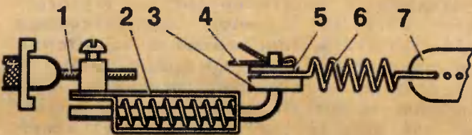
Рис. 2. Крепление троса к рычагу дроссельной заслонки: 1 — трос; 2 — компенсатор; 3 — рычаг дроссельной заслонки; 4 — шплинт; 5 — шайба; 6 — пружина; 7 — полоса.
