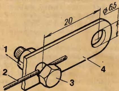
Рис. 1. Наконечник троса: 1 — гайка М8; 2 — трос; 3 — винт М8 с отверстием диаметром 2 мм; 4 — пластина.
